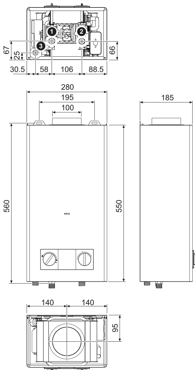
fig. 19 - Medidas y conexiones CAMI 6
