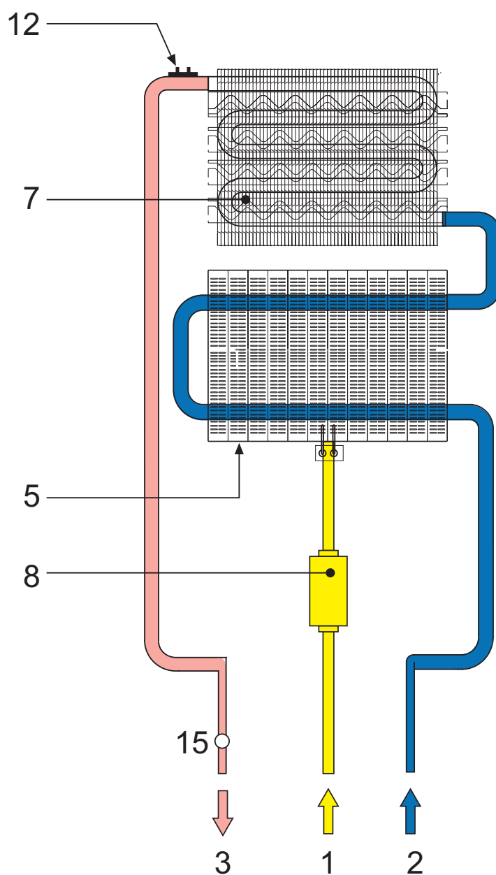
fig. 23 - Circuito idraulico
