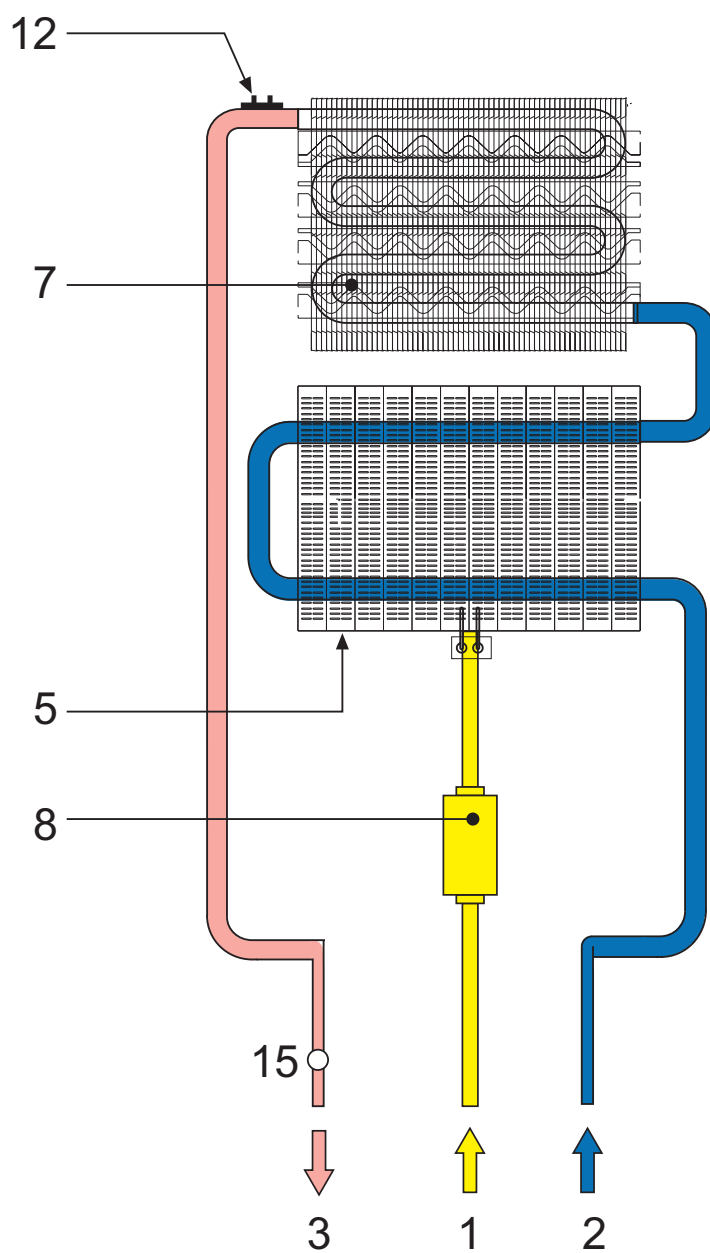
fig. 23 - Circuito hidráulico
