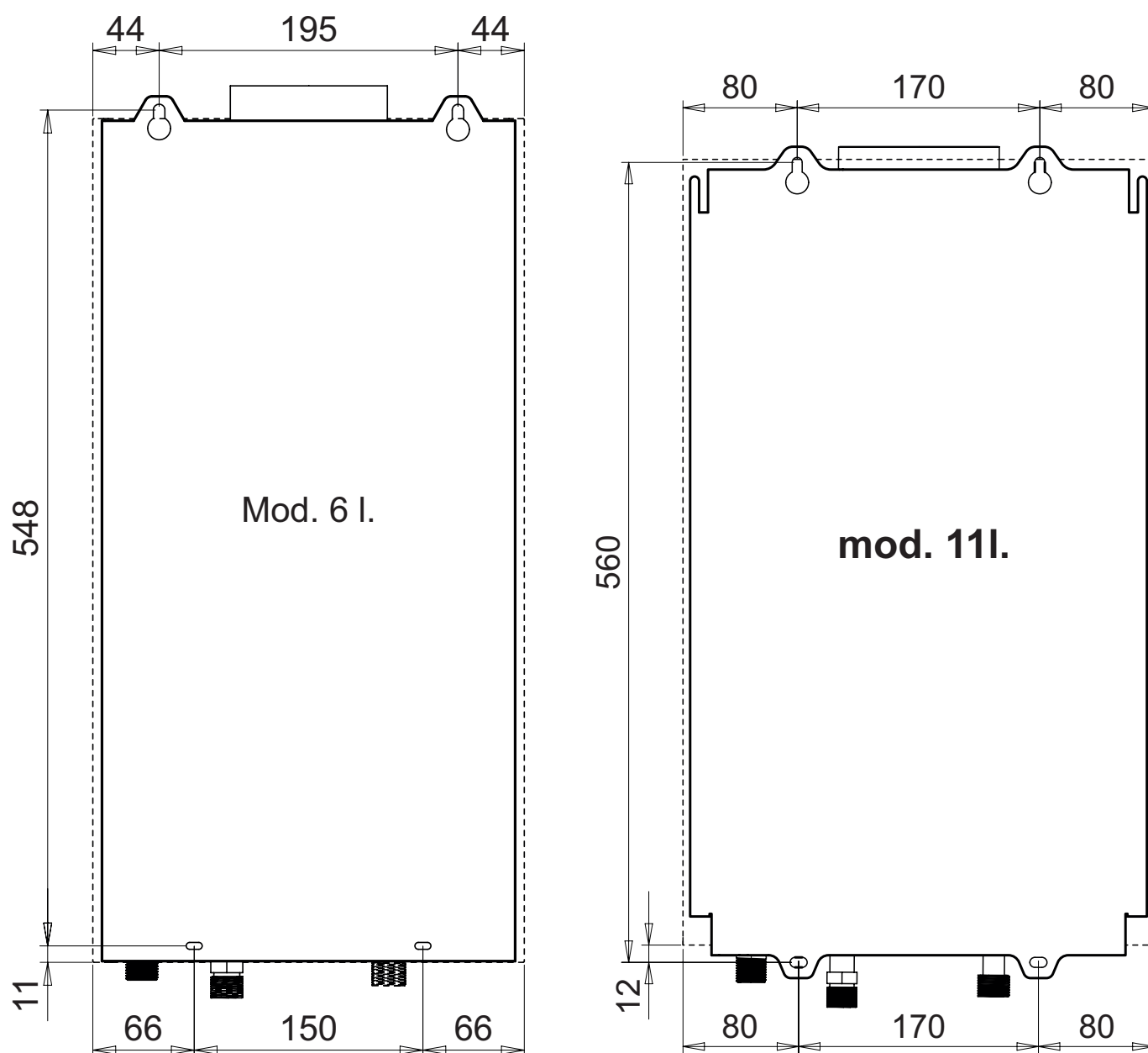
fig. 6 - Assembly template
